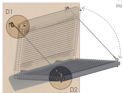
Aggancio fissato alla struttura con moschettone per fissare il letto nella posizione chiusa
